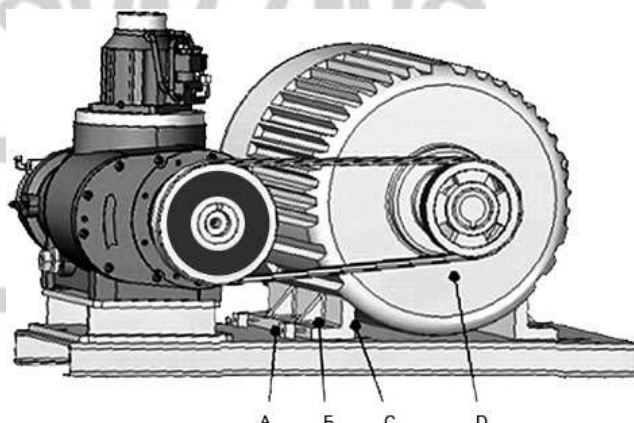
A - Регулировочный болт B - Болт крепления C - Направляющая пластина основания двигателя D - Электромотор
